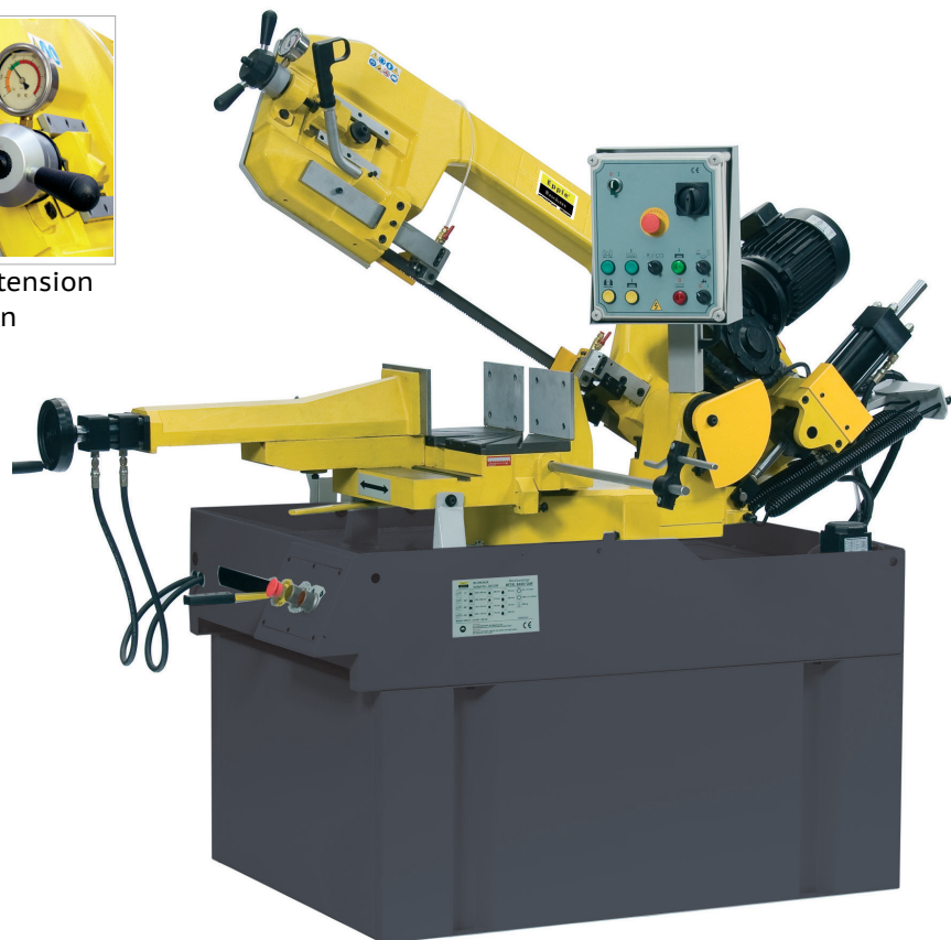
FIG.: BS 350 DGHF
